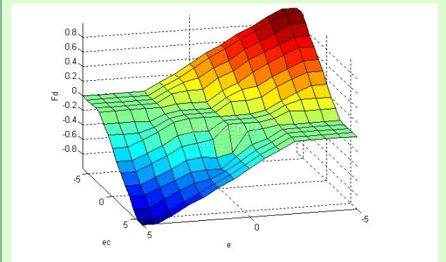
Fuzzy Controller
